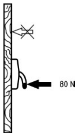
Porte sans pression
