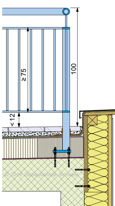
Fig. 10: Hauteur des éléments de protection et ouvertures dans les éléments de protection Une isolation résistant à la compression dans la zone de la console, env. 40 x 40 cm, comme fond solide pour l'étanchéité à polymère liquide est recommandée.
