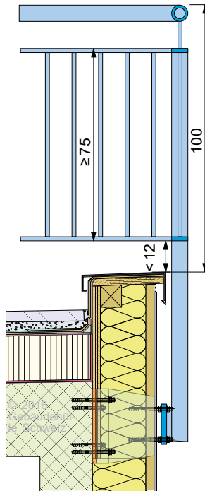
Fig. 8: Éléments en saillie, accessibles, couronnement de mur
