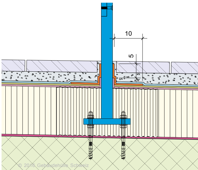
Fig. 15: Console de garde-corps ne permettant pas l'infiltration d'eau avec surface adhésive de 5 cm directement sur le montant. Une isolation thermique résistante à la compression dans la zone de raccordement sous la surface adhésive en PL est recommandable.
