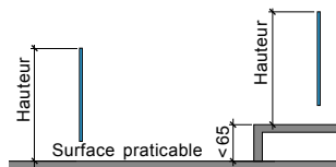
Fig. 2: Hauteur de l'élément de protection
