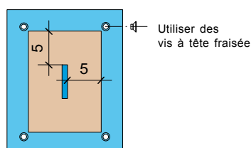
Fig. 13: Surface adhésive pour PL, minimum 5 cm, sans traversées
