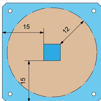
Fig. 12: Surface adhésive pour lés d'étanchéité en bitume polymère (LBP), minimum 12 cm, sans traversées
