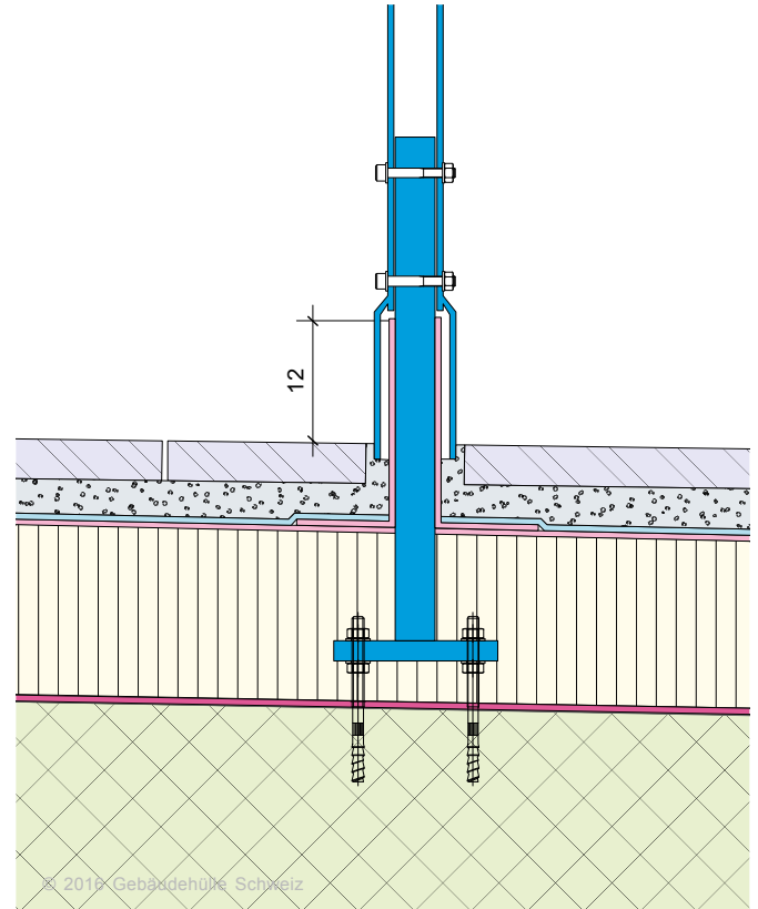
Fig. 17: Raccordement d'étanchéité de console de garde-corps ouvert en haut avec garniture plastique et élastomère. Montant de garde-corps avec cloche couvrant le raccordement de l'étanchéité.
