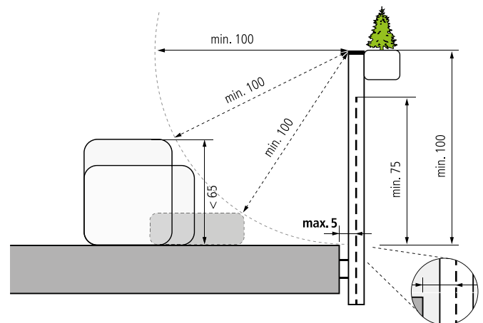
Fig. 20: Distance entre les bacs à plantes, bancs et meubles et le garde-corps, voir la recommandation bfu (illustration bfu)
