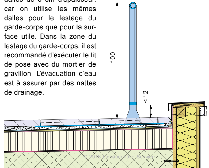
Fig. 19: Garde-corps système avec lestage par la couche d'usure. Tenir compte des exigences système.
