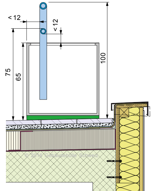
Fig. 9: Bac à plantes comme partie de l'élément de protection. La résistance à la compression (charge permanente) de l'isolation thermique doit être calculée. Recommandation bfu: Hauteur des bacs à plantes: 75 cm
