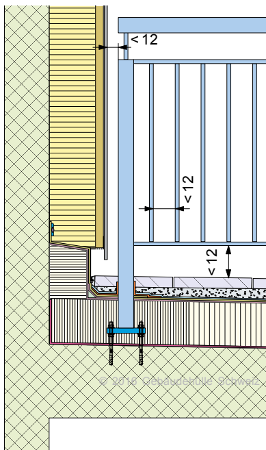
Fig. 10: Hauteur des éléments de protection et ouvertures dans les éléments de protection Une isolation résistant à la compression dans la zone de la console, env. 40 x 40 cm, comme fond solide pour l'étanchéité à polymère liquide est recommandée.
