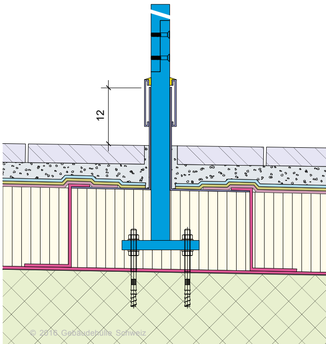
Fig. 16: Raccordement d'étanchéité de console de garde-corps ouvert en haut, surfaces adhésives voir Fig. 12 et manchon de bande de recouvrement autour du montant. Le colmatage de la surface adhésive peut être fait de manière linéaire sur toutes les consoles ou individuellement.
