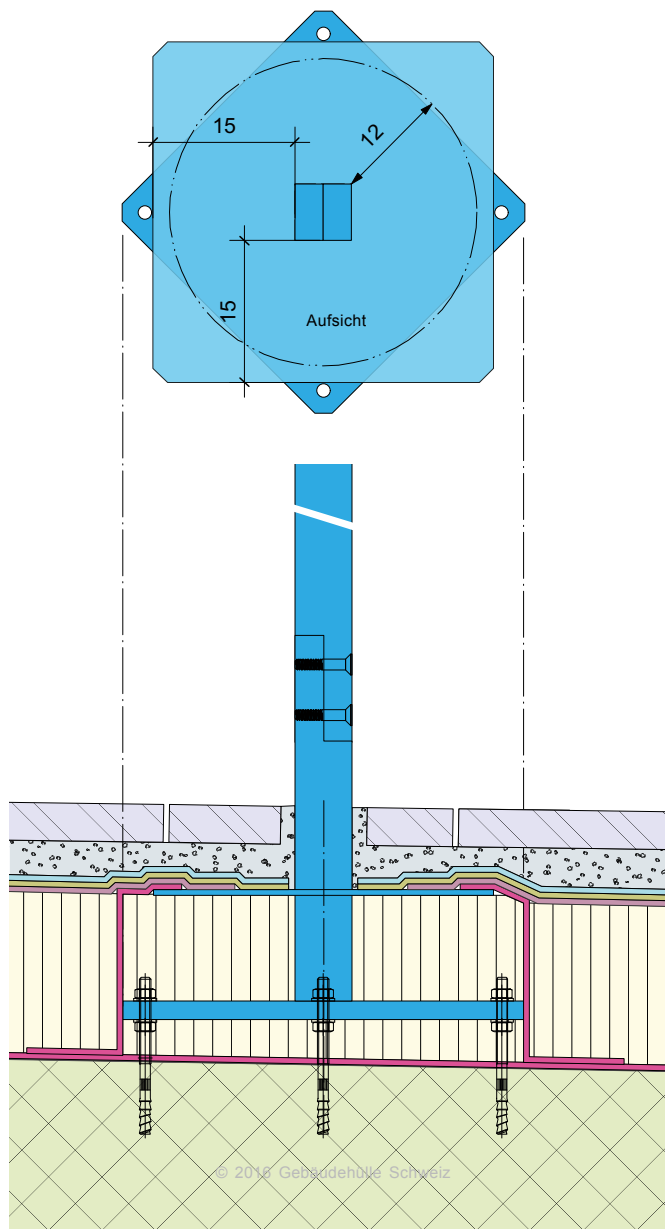
Fig. 14: Console de garde-corps avec surface adhésive bitumineuse selon Fig. 12. Flasque de montage inférieur tourné de 45° pour qu'il prenne le moins de place possible. Le colmatage de la surface adhésive peut être fait de manière linéaire sur toutes les consoles ou individuellement.
